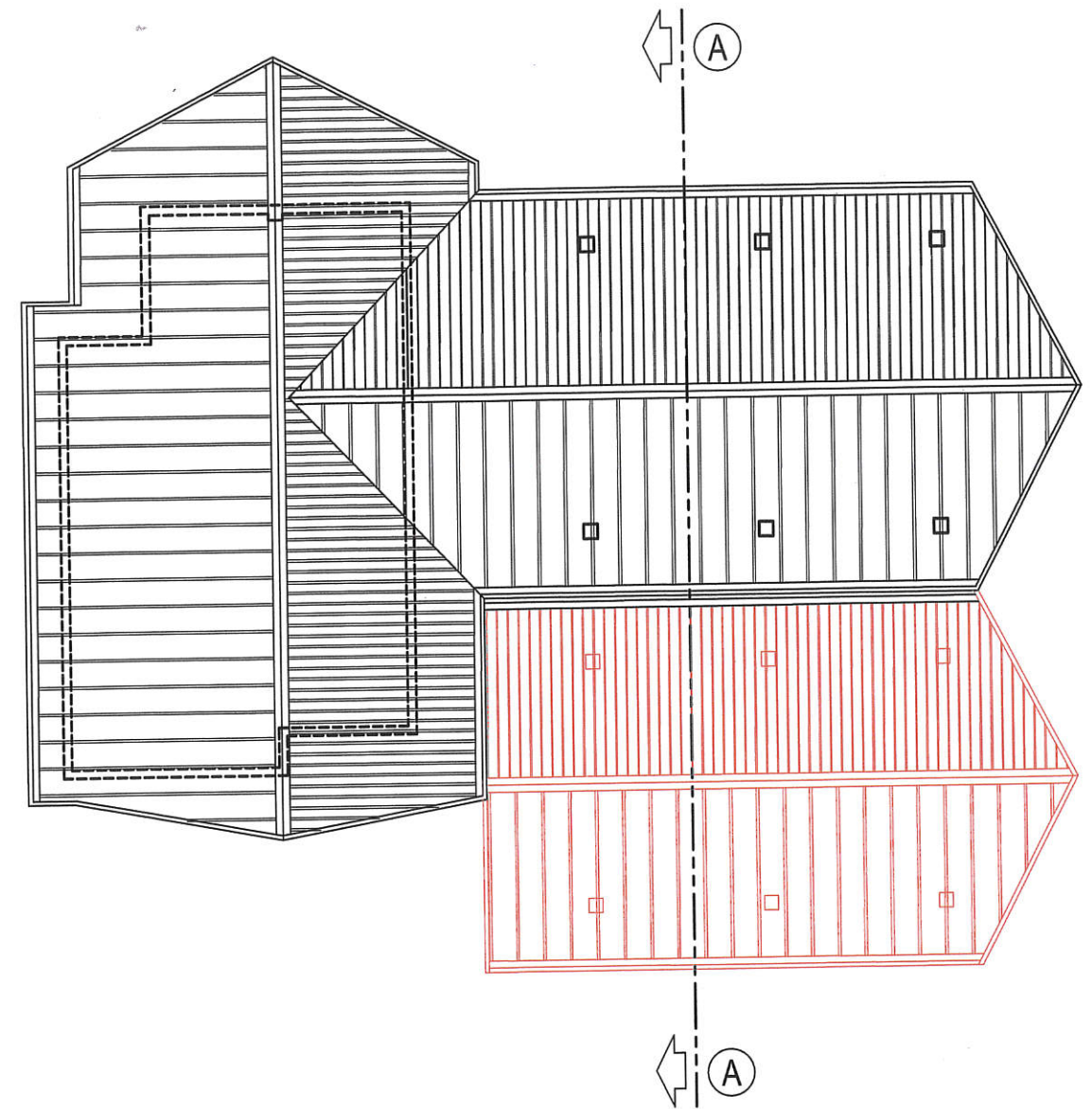
sezione A:A
